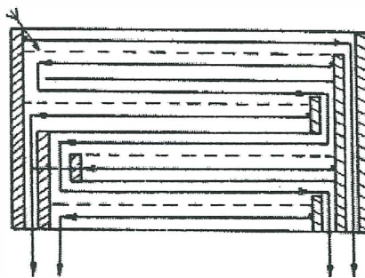
Dibujo 9. Corte de un "plansichters" en trituración.
