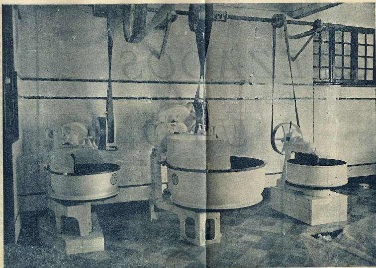
Amasadora-Batidora
