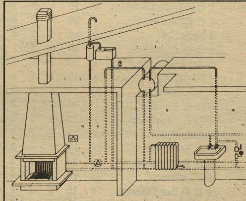
PUEDEN DOTAR DE CALEFACCIÓN CENTRAL A SU VIVIENDA
